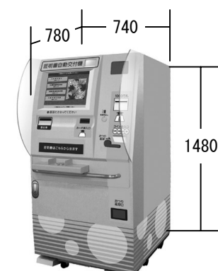
外観寸法図 (単位: mm) 突起部除く
